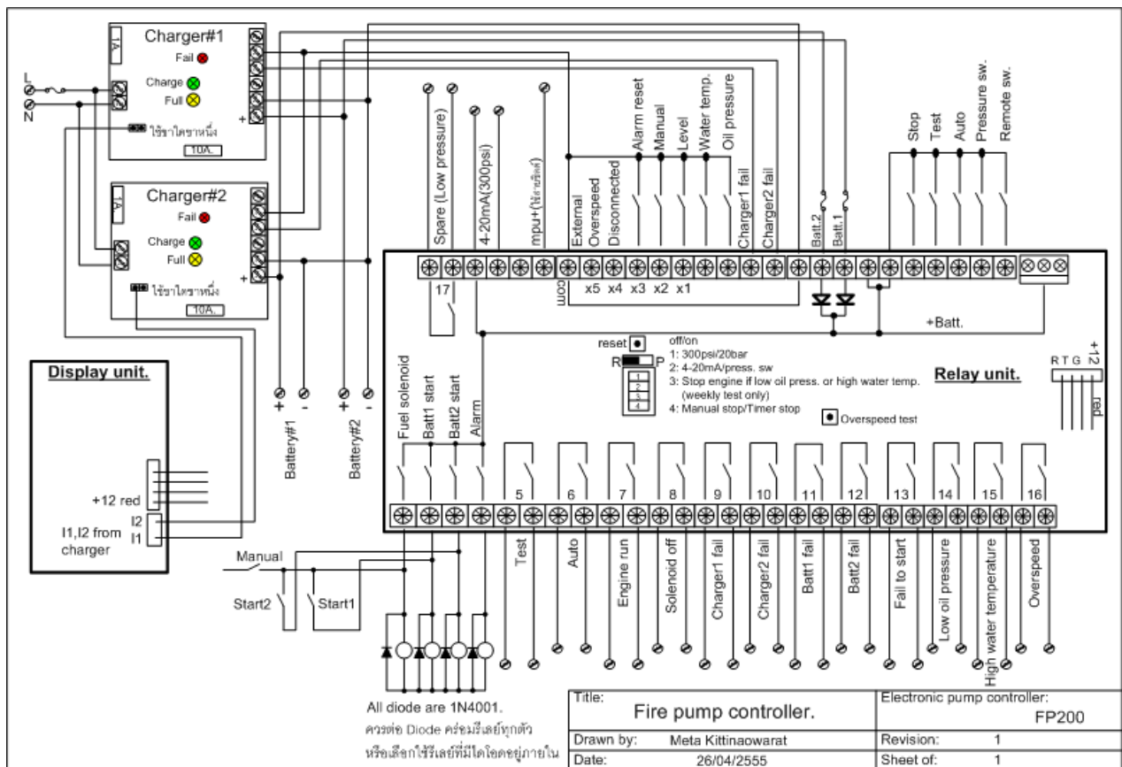
ตัวอย่างแบบ wiring.
